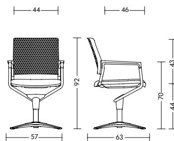
mer60 mit Armlehne with arm supports 11 kg
