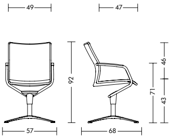
cie90 mit Armlehne with arm supports 13 kg
