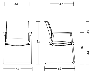
mer56 mit Armlehne with arm supports 9 kg
