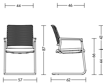
mer46 mit Armlehne with arm supports 9 kg
